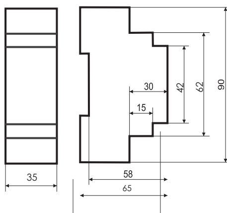
Рис.4 Габаритные размеры.
