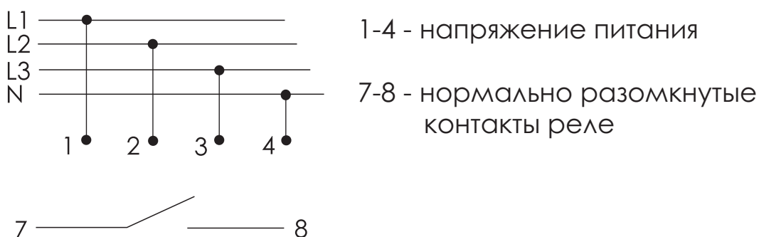
Рис.2 Назначение контактов.
